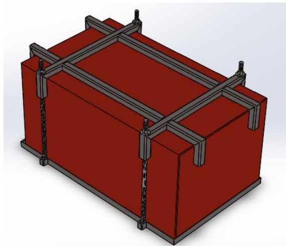
Figura 2. Montaje contenedor
