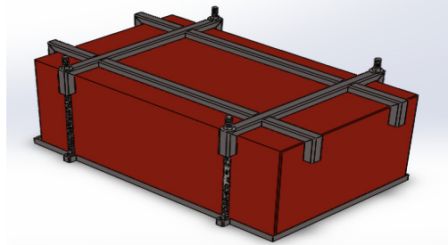
Figura 2. Montaje contenedor
