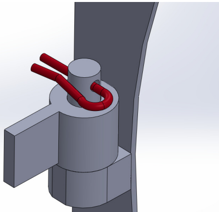
Ejemplo de sujeción realizado con chaveta "R"
