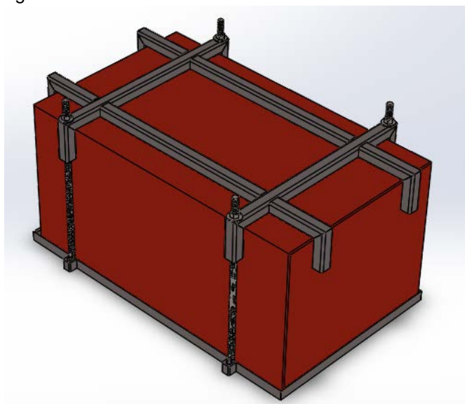
Figura 2. Montaje contenedor
